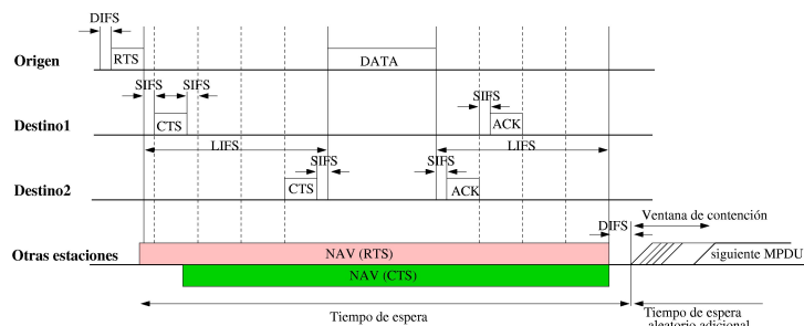
Figura 2: Mecanismo RTS CTS ACK en LLRB
