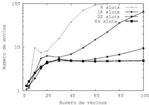
Figura 4: Número de envíos necesarios hasta asentar todas las tramas
