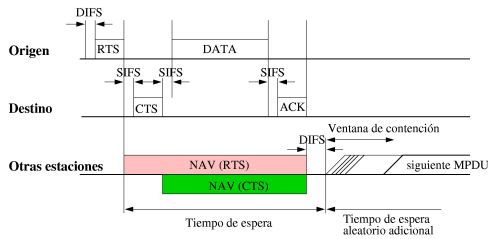
Figura 1: Mecanismo RTS CTS ACK
