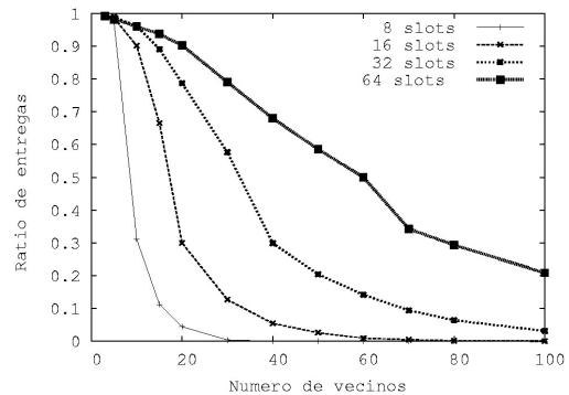
Figura 3: Ratio de paquetes entregados en el primer envío
