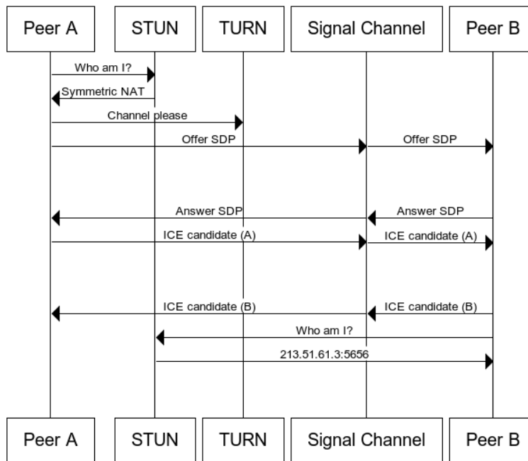
Figura 3.4: Diagrama de establecimiento de sesión en WebRTC con STUN y TURN
