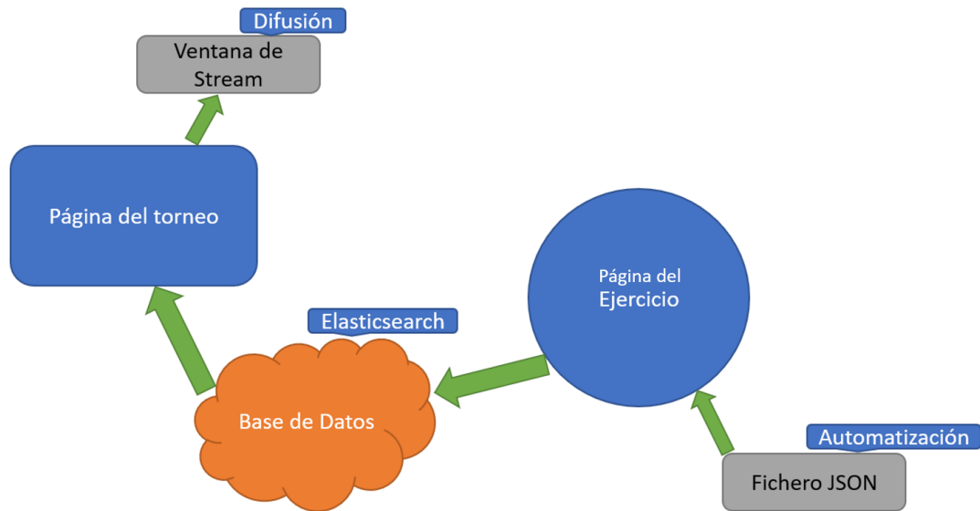
Figura 5.1: Diseño de la infraestructura de los torneos de ranking
