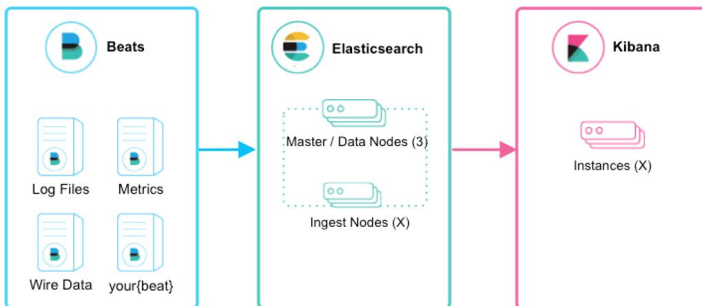
Figura 3.1: Arquitectura de Elasticserch, Beats y Kibana
