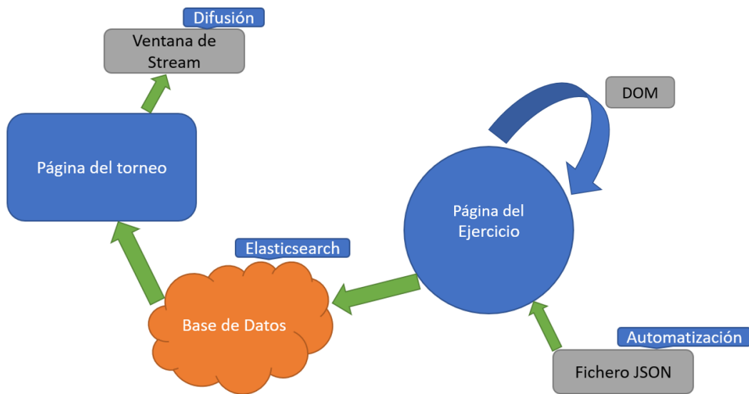
Figura 5.2: Diseño de la infraestructura de los torneos de enfrentamientos
