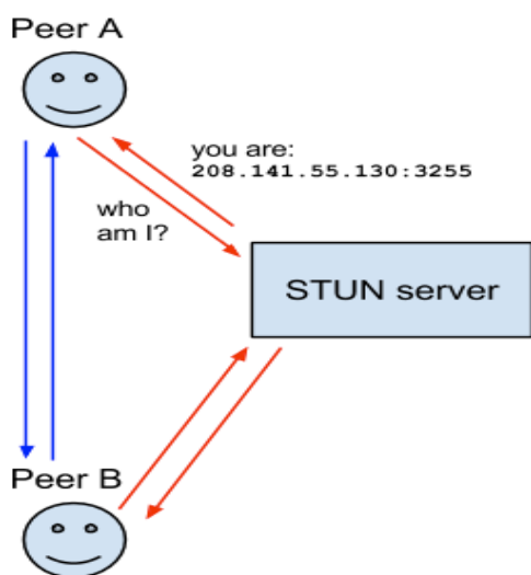
Figura 3.2: Protocolo STUN
