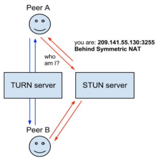
Figura 3.3: Protocolo TURN
