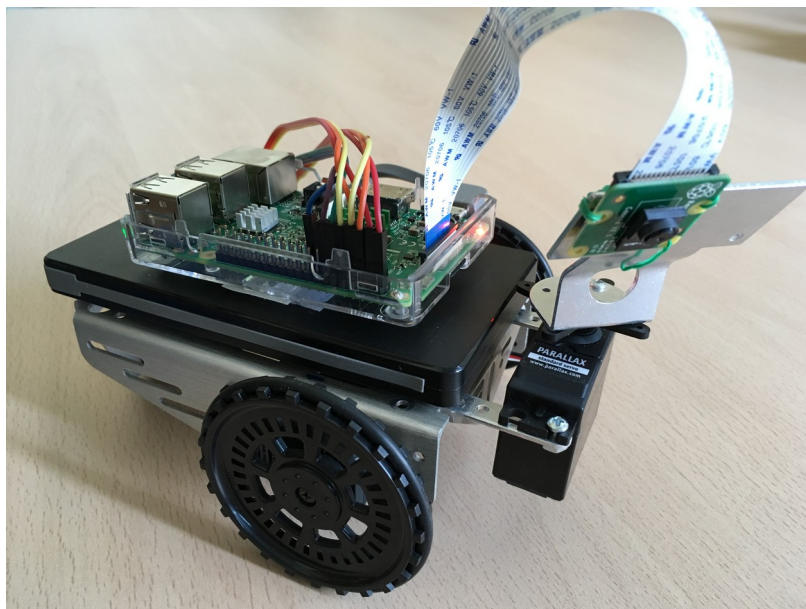
Figura 1. PiBot con su PiCamera montada en una unidad panorámica
