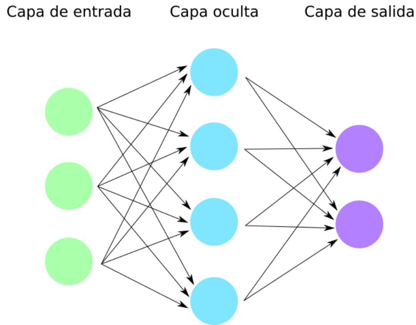
Figura 3.9: Red neuronal de tres capas y ocho neuronas.
