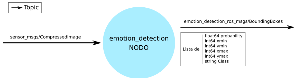
Figura 4.10: Esquema general del paquete de ROS.
