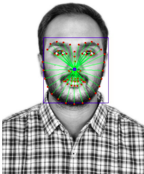
Figura 4.3: Distancias entre puntos faciales del artículo [Rohith Raj S, Pratiba D, 2020].
