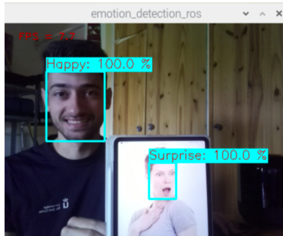
Figura 4.12: Ejemplo del sistema en ROS detectando las emociones de dos caras.
