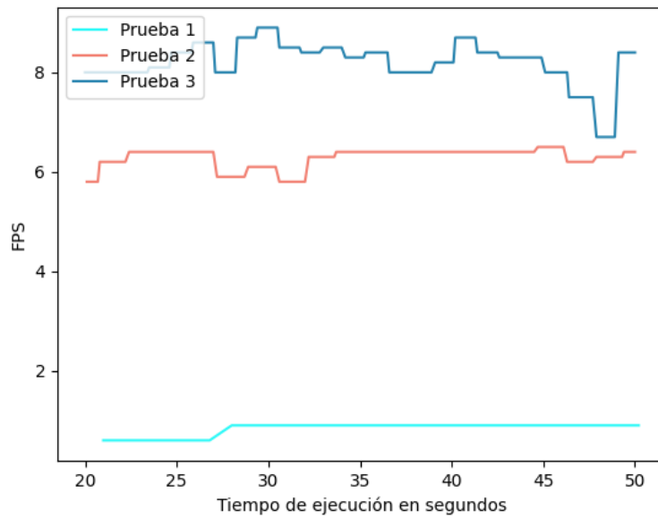
Figura 5.1: Comparativa de las tres pruebas de rendimiento de dlib.
