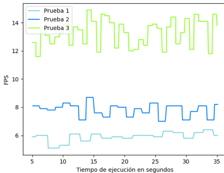
Figura 5.3: Comparativa de las tres pruebas de rendimiento de MediaPipe.
