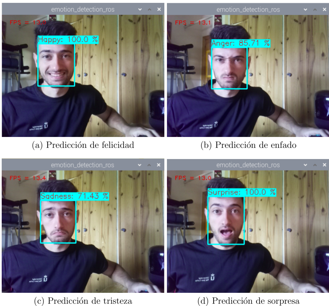
Figura 4.11: Ejemplos de la ventana gráfica del sistema de detección de emociones funcionando en ROS.
