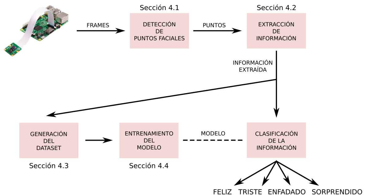
Figura 4.1: Método de detección de emociones.
