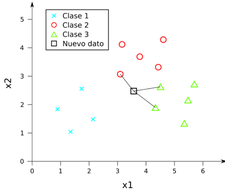
Figura 3.8: Ejemplo de KNN con k = 3 .
