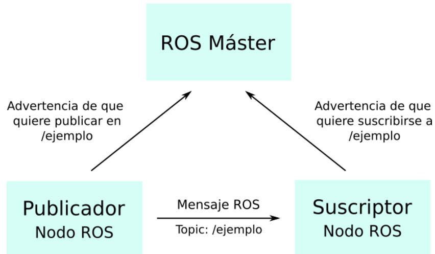
Figura 3.12: Esquema simple de una comunicación publicador-suscriptor en ROS.
