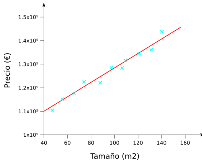
Figura 1.13: Ejemplo de regresión lineal. Predicción del precio de la vivienda.
