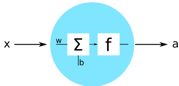
Figura 3.10: Ejemplo del interior de una neurona de una entrada, donde x es la entrada y a es la salida.
