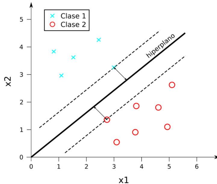
Figura 3.7: Hiperplano de separación óptimo entre los datos de dos clases.
