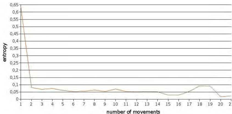
Fig. 10. Bel entropy
